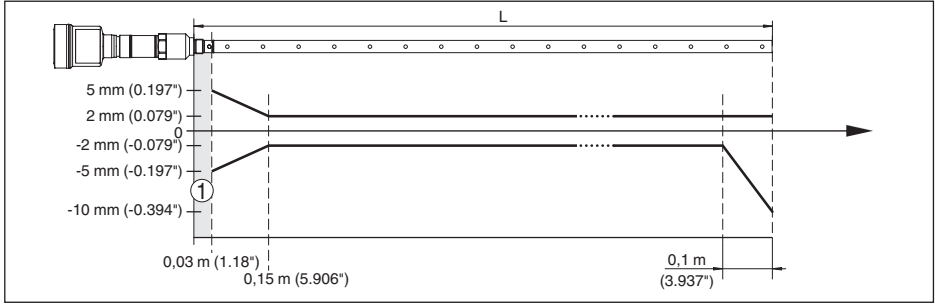
插图 19: 在介质“水”中同轴型的测量偏差 NivoGuide 8200 (测量长度至 1.5 m/4.92 ft)
