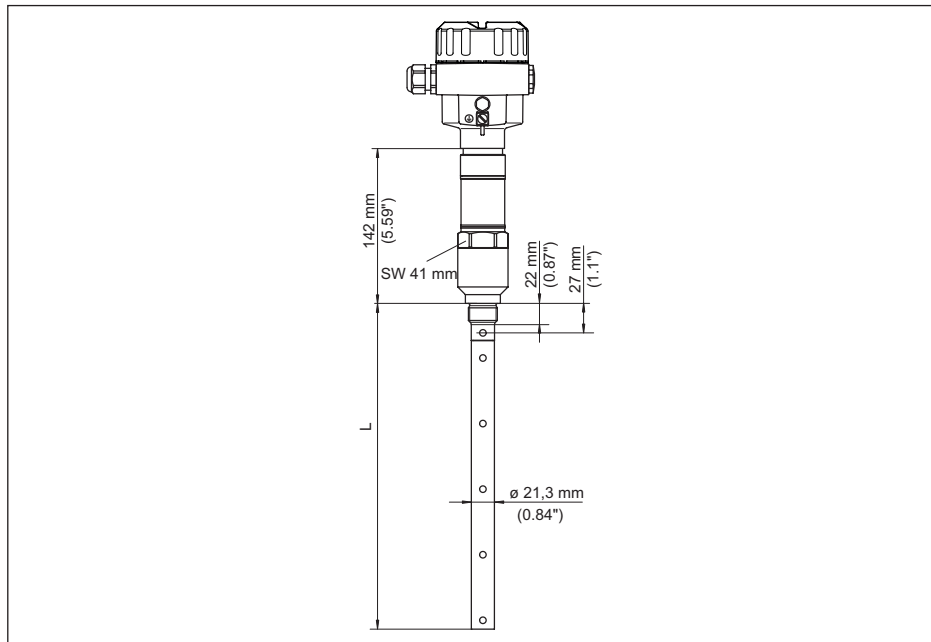
插图. 28: NivoGuide 8200, 带螺纹的同轴型 (-20 ... +250 °C/-4 ... +482 °F)
