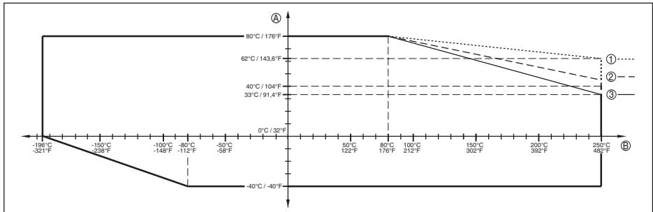
插图. 23: 环境温度 - 过程温度, 标准型
