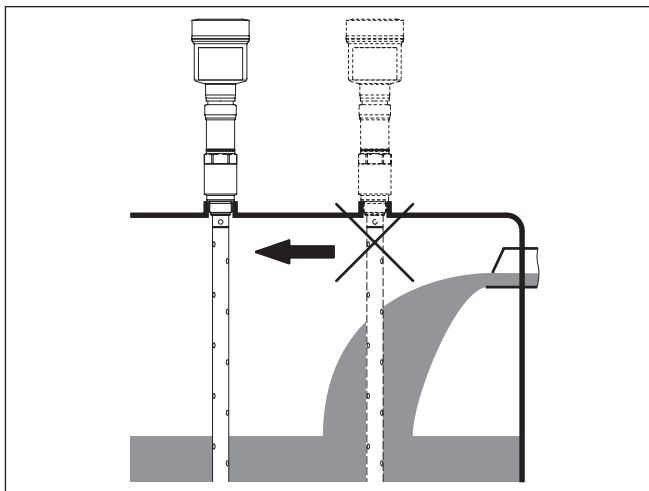
插图. 5: 流入介质时安装传感器
