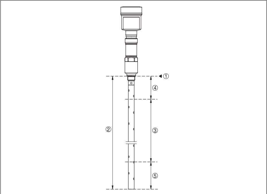
插图. 18: NivoGuide 8200 的测量范围
