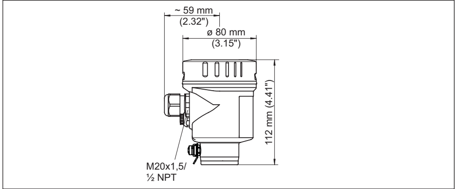
插图. 26: 采用保护等级达 IP 66/IP 68 (0.2 bar) 的壳体型式, (内装显示和调整模块后, 壳体高度增加了 9 mm/0.35 in)
