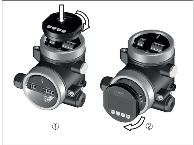
插图. 13: 将显示和调整模块装到双腔式壳体上
