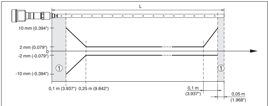
插图 21: 在介质“油”中同轴型 NivoGuide 8200 的测量偏差 (测量长度至 1.5 m/4.92 ft)
