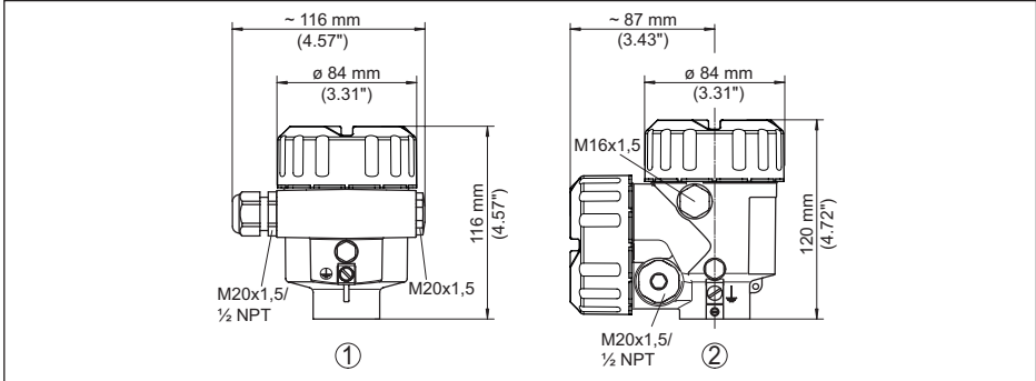
插图. 24: 采用保护等级达 IP 66/IP 68 (0.2 bar) 的壳体型式, (内装显示和调整模块后, 壳体高度增加了 9 mm/0.35 in)
