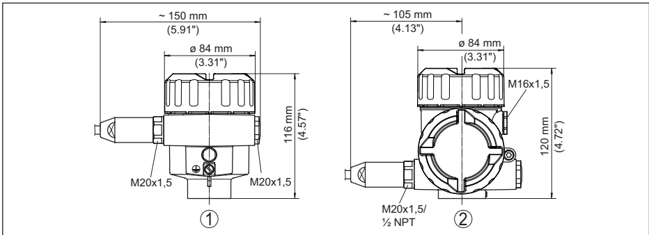
插图. 25: 采用保护等级达 IP 66/IP 68 (1 bar) 的壳体型式, (内装显示和调整模块后, 壳体高度增加了 9 mm/0.35 in)
