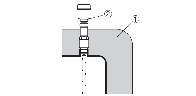
插图. 7: 将仪表安装在绝缘容器上。
