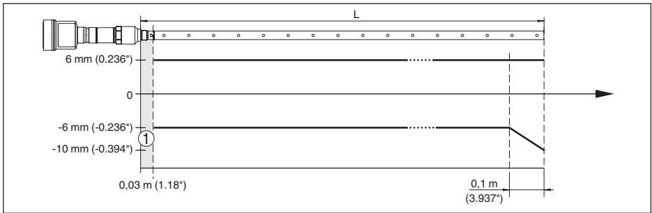
插图 20: 在介质“水”中同轴型 NivoGuide 8200 的测量偏差 (测量长度至 6 m/19.69 ft)
