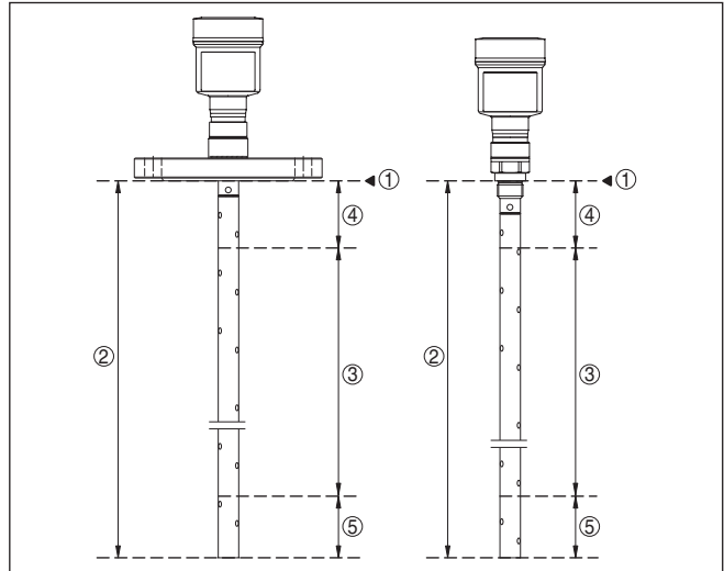
Abb. 8: Messbereiche - NivoGuide 8100
