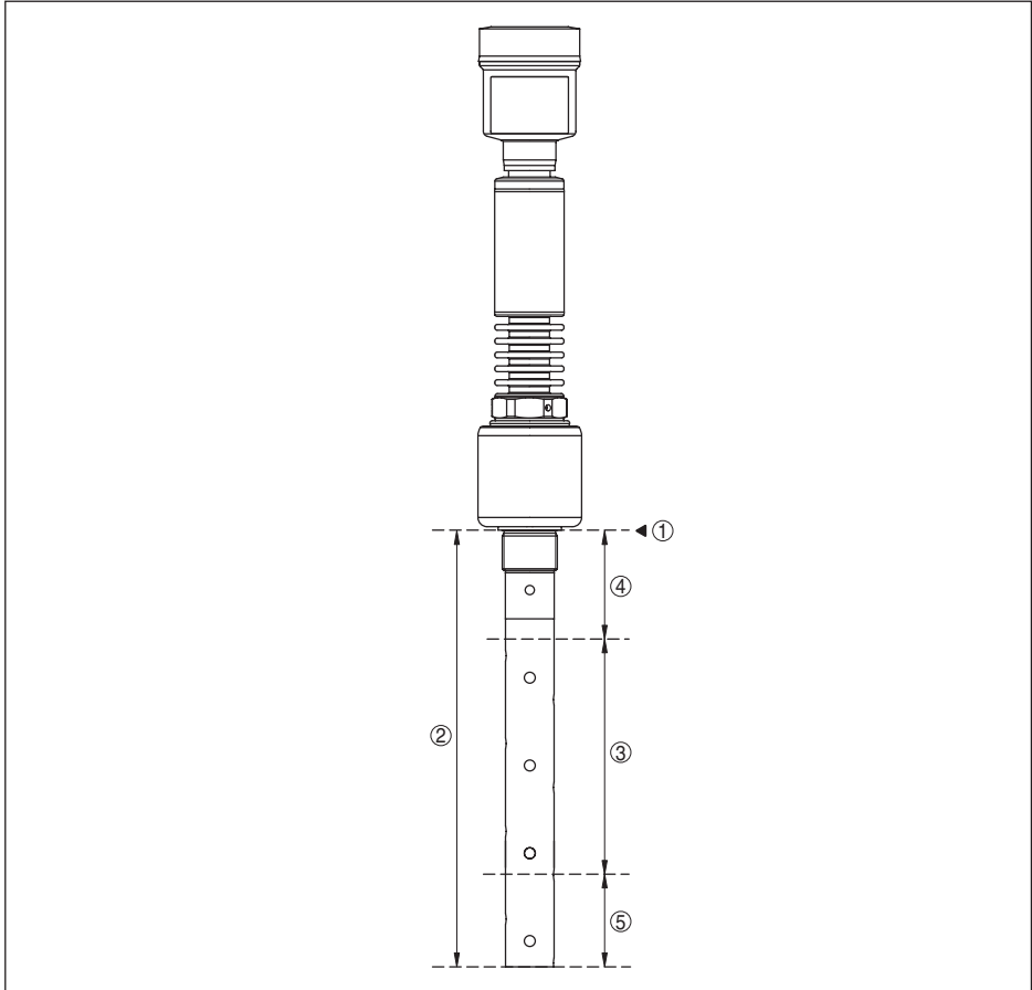
Fig. 24: Rangos de medida - NivoGuide 8200
