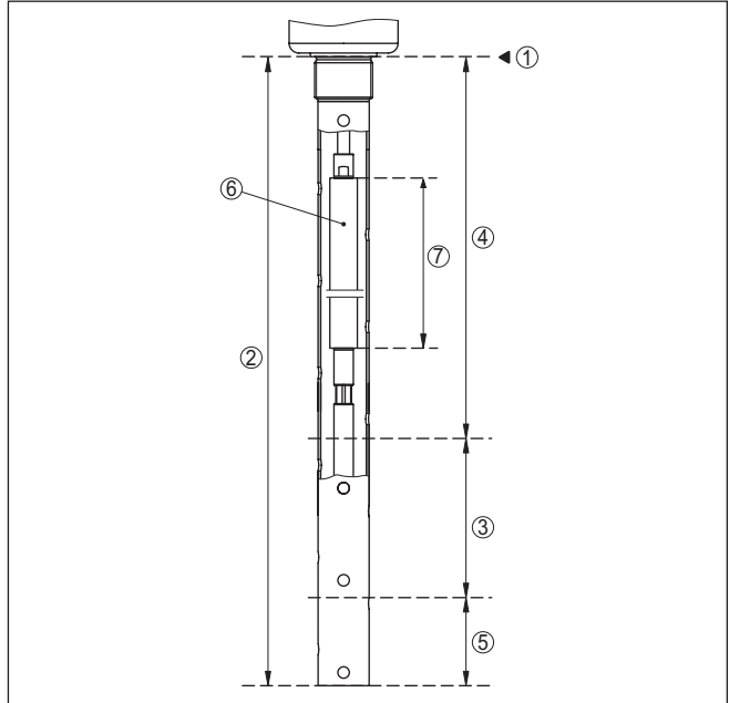
Fig. 8: Rangos de medición - NivoGuide 8200 con compensación de vapor
