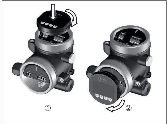
Fig. 14: Empleo del módulo de visualización y configuración en carcasa de dos cámaras
