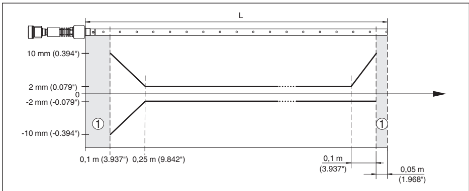
Fig. 22: Error de medición NivoGuide 8200 en versión coaxial en producto aceite (longitud de medición hasta 1,5 m/4.92 ft)
