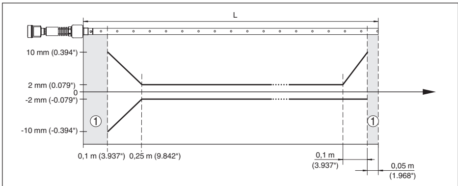
Fig. 27: Error de medición NivoGuide 8200 en versión coaxial en producto aceite (longitud de medición hasta 1,5 m/4.92 ft)
