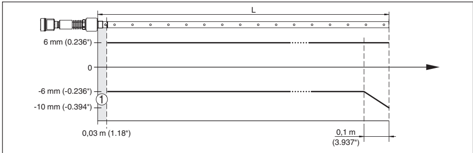
Fig. 26: Error de medición NivoGuide 8200 en versión coaxial en producto agua (longitud de medición hasta 6 m/19.69 ft)
