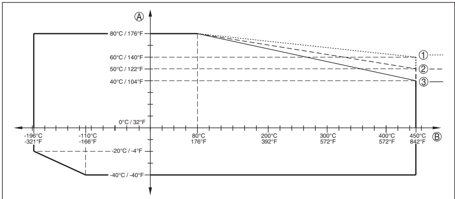
Fig. 30: Temperatura ambiente - Temperatura de proceso, versión estándar
