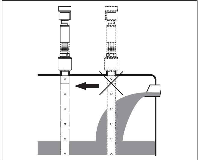
Fig. 5: Montaje del sensor en flujo de entrada de producto
