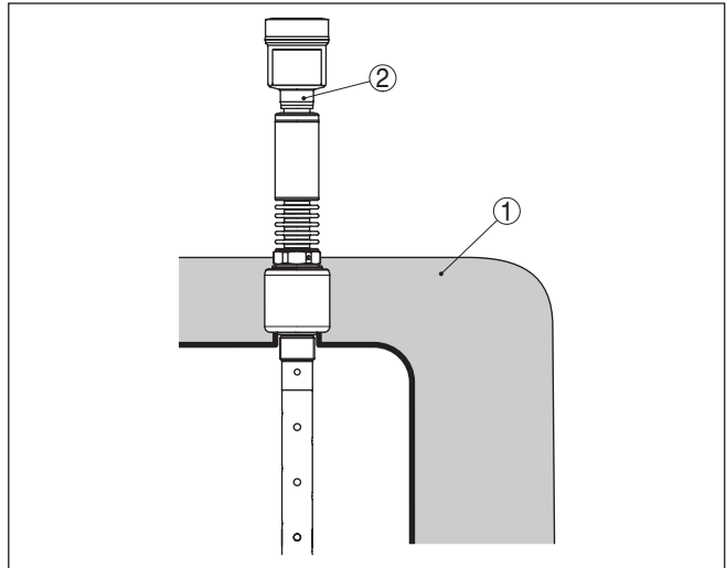
Fig. 7: Montaje del equipo con depósito aislado
