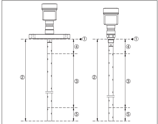
插图. 8: NivoGuide 8100 的测量范围
