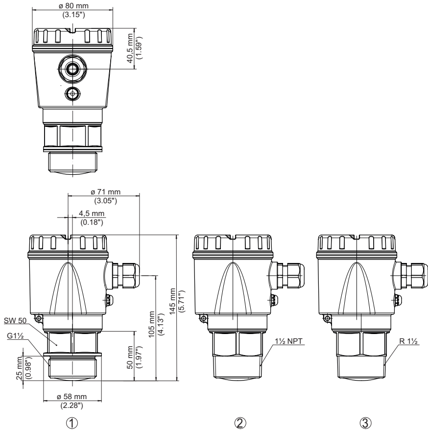
Рис. 7: Размеры NivoRadar 7200
