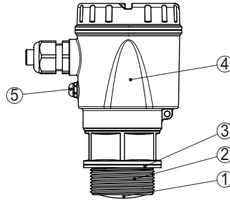
Рис. 1: Компоненты NivoRadar 7200
