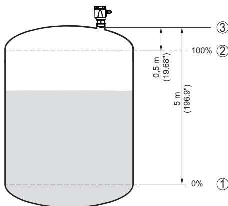
Рис. 23: Пример выполнения Установки Min./Max.
