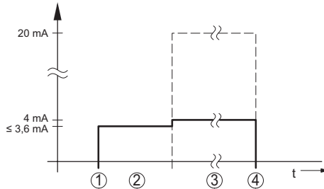
Рис. 5: Время запуска и выдача измеренного значения
