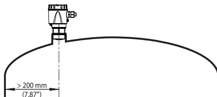
Рис. 10: Монтаж бесконтактного микроволнового уровнемера на округлой крыше емкости
