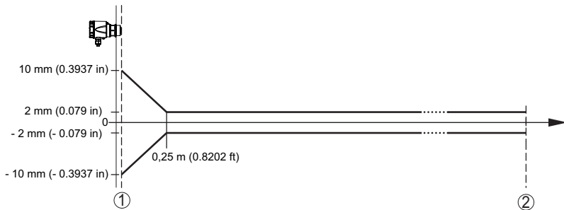
Рис. 6: Погрешность измерения при нормальных условиях 2)
