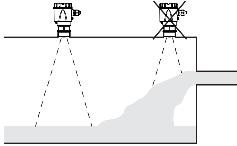
Рис. 12: Монтаж бесконтактного микроволнового уровнемера при втекающей среде
