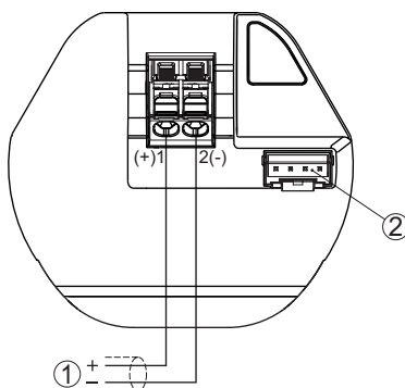
Рис. 19: Отсек подключения NivoRadar 7200
