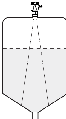
Рис. 11: Монтаж бесконтактного микроволнового уровнемера на емкостях с коническим дном
