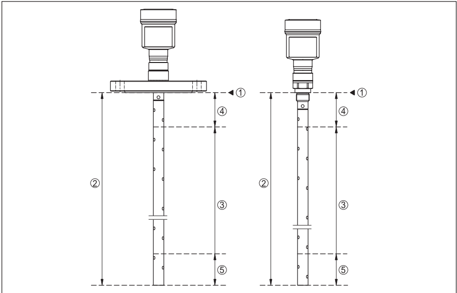
插图 25: NivoGuide 8100 的测量范围
