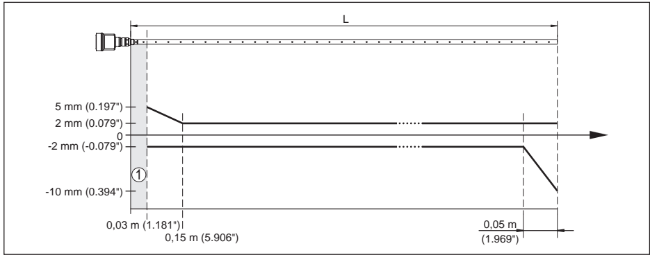
插图. 26: 同轴型 NivoGuide 8100 在介质“水”中的测量偏差
