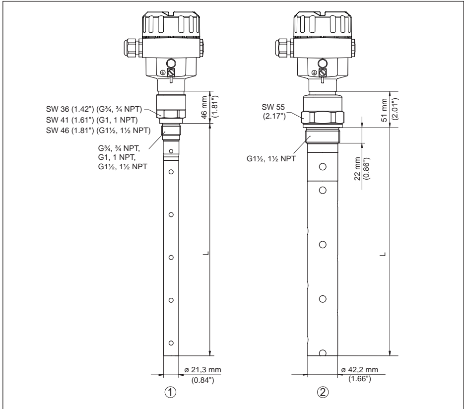
插图. 32: NivoGuide 8100, 螺纹型
