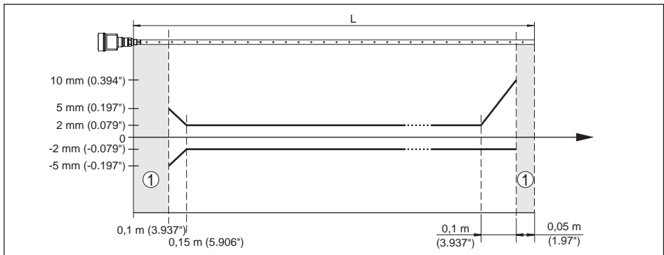
插图. 27: 同轴型 NivoGuide 8100 在介质“油”中的测量偏差
