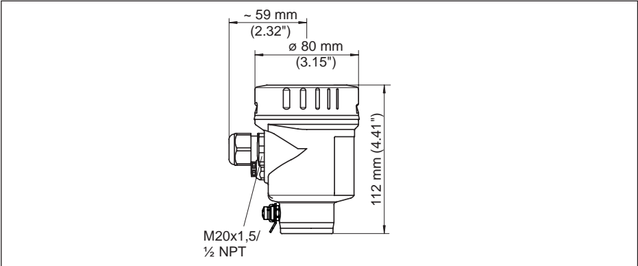
Fig. 41: Variante de carcasa en grado de protección IP 66/IP 68; (0,2 bar), (con módulo de visualización y configuración integrado aumenta la altura de la carcasa en 9 mm/0.35 in)
