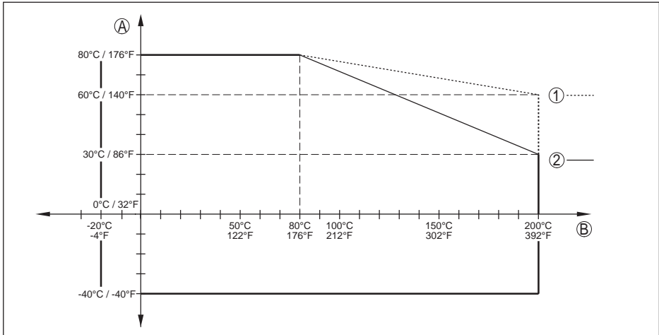
Fig. 39: Temperatura ambiente - Temperatura de proceso, versión con adaptador de temperatura
