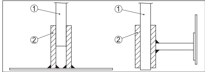
Fig. 9: Fijar la sonda de medición
