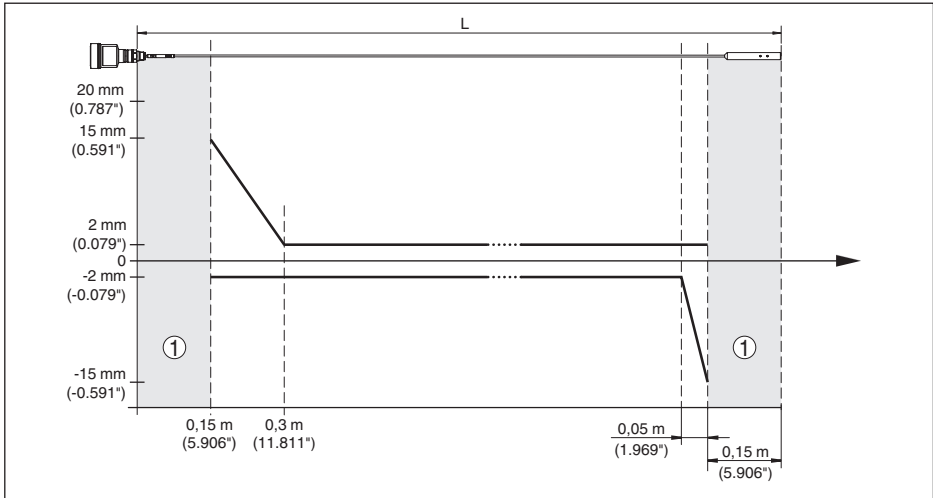
Fig. 35: Error de medición NivoGuide 8100 en versión cableada ( \varnothing 4 mm/0.157 in), en aceite
