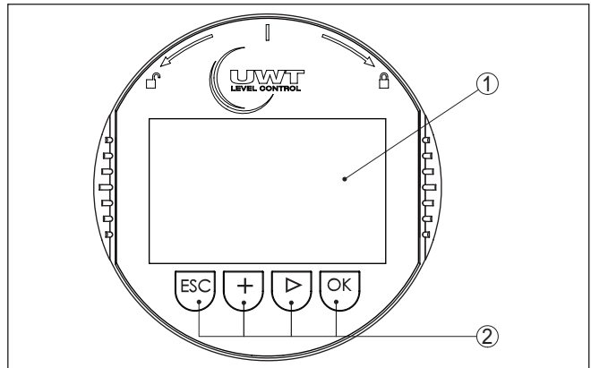
Fig. 16: Elementos de indicación y ajuste
