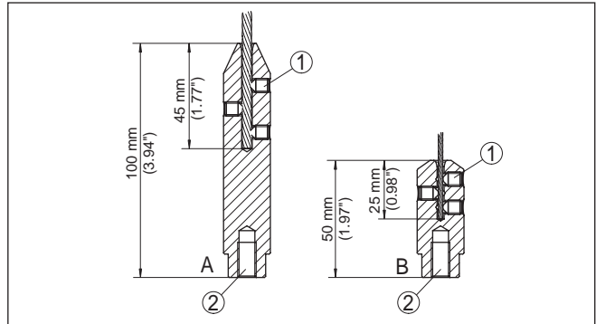
Fig. 29: Reducción de la celda de medida cableada
