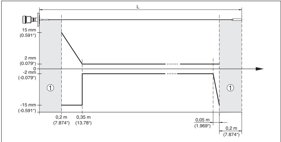
Fig. 37: Desviación NivoGuide 8100 en versión de cable (ø 4 mm/0.157 in, revestida de PFA) en aceite 1 Distancia de bloqueo (En esta zona no es posible ninguna medición) L Longitud de la sonda de medición
