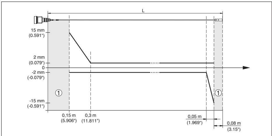
Fig. 34: Error de medición NivoGuide 8100 en versión cableada (ø 2 mm/0.079 in), en aceite
