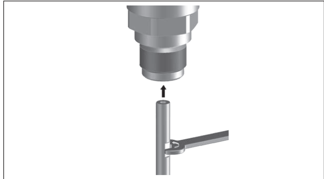
Fig. 28: Cambiar cable de medición y varilla de medición
