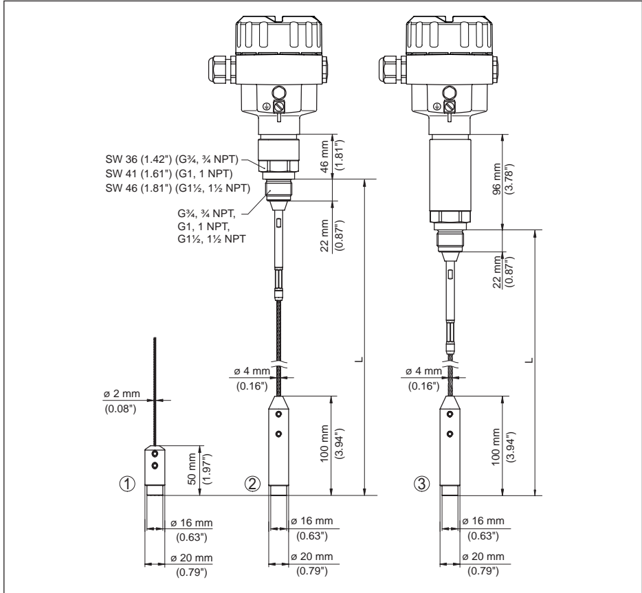
Fig. 42: NivoGuide 8100, versión roscada con peso tensor (todos los pesos tensores con rosca M8 para tornillo de cáncamo)
