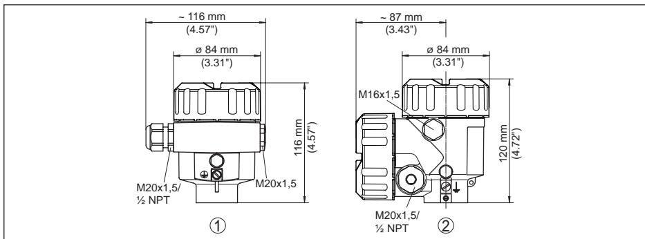
Fig. 40: Variante de carcasa en grado de protección IP 66/IP 68; (0,2 bar), (con módulo de visualización y configuración integrado aumenta la altura de la carcasa en 9 mm/0,35 in)
