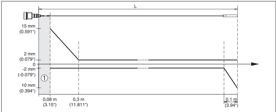
Fig. 33: Error de medición NivoGuide 8100 versión cableada en agua
