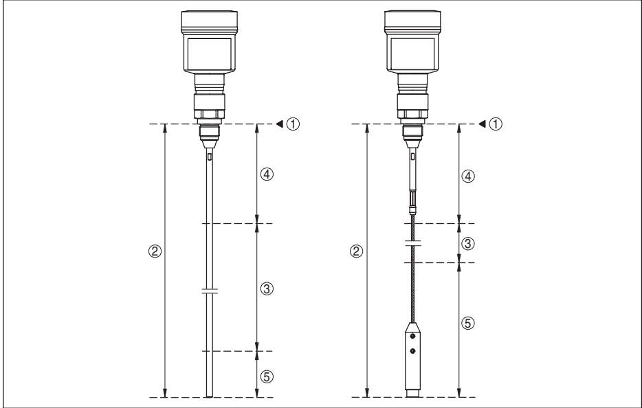
Fig. 30: Rangos de medida - NivoGuide 8100
