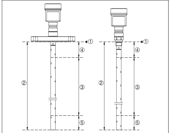
Fig. 8: Plages de mesure - NivoGuide 8100
