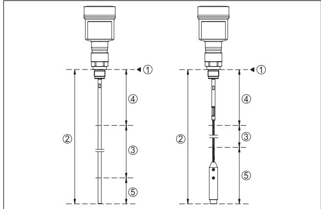
Fig. 11: Rangos de medida - NivoGuide 8100
